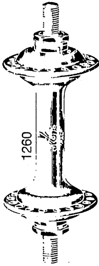
1250 NUOVO TIPO SMALL FLANGE CAMPAGNOLO SOLID SPINDLE HUBS
